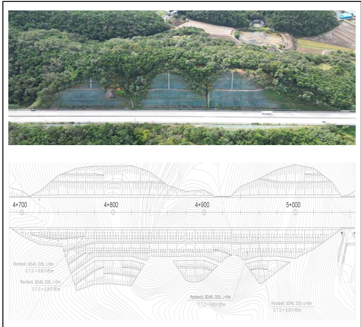
【그림 46.14】 영천절토46 검토대상 비탈면구간
